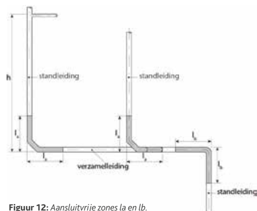
Figuur 12: Aansluitvrije zones l_a en l_b .
