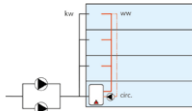
Figuur 6: Meerdere drukgroepen, warmtapwaterbereider in elke drukgroep.
