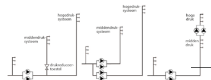
Figuur 1: Meerdere drukzones door toepassing van drukreductietoestel of meerdere drukverhogingsinstallaties.
