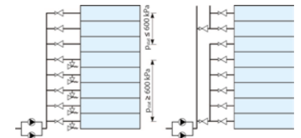
Figuur 3: Grote hoogte met een enkele drukverhogingsinstallatie door gebruik van veiligheidsventielen of in serie geschakelde drukreductietoestellen.
