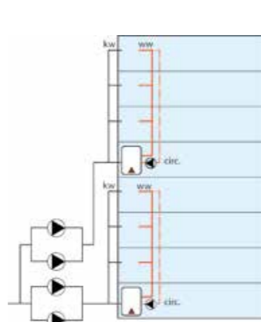
Figuur 7: Eén of meerdere drukgroepen, lokale warmtapwaterbereiders
