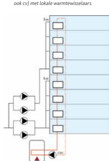
Figuur 8: Eén of meerdere drukgroepen, centrale warmtapwaterbereiding (meestal ook cv) met lokale warmtewisselaars.
