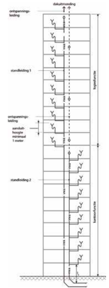
Figuur 9: Gescheiden standleidingen per gebouwfunctie.
